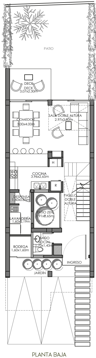
PLANTA BAJA
